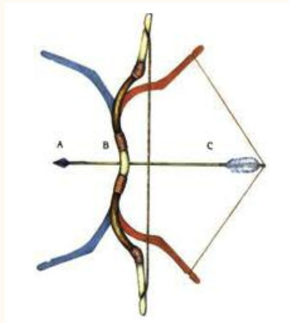
복합궁, 조립식활의 작동원리
